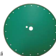
Tăiere uscată Prindere: Ø 25,4 mm Segment continuu Turbo Aplicații: granit, marmură, beton.
