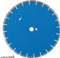
Tăiere umedă și uscată Prindere: Ø 25,4 mm Nr. segmenti: 36/40 Aplicații: beton, pavele din beton.
